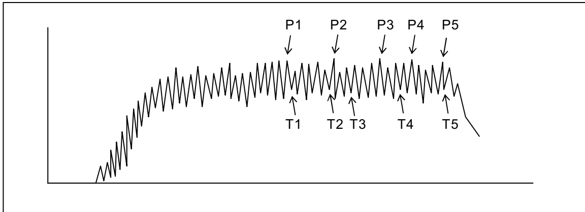
Figure 2a – Enregistrement de la tension du corps en polarité positive
